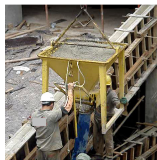
Fotos ilustrativas – Sistema duplo de segurança - Exemplo do equipamento em campo
